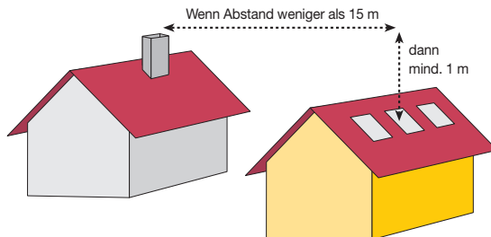
Mindesthöhe von Kaminmündungen in Abhängigkeit der Entfernung zum benachbarten Wohngebäude.
